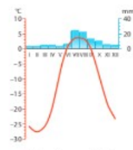
Klimatogram dla Barrow na Alasce (Stany Zjednoczone, Ameryka Północna).
